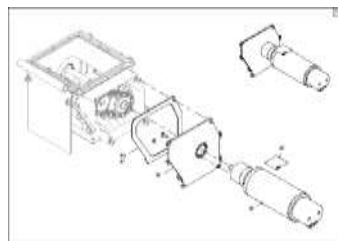
ЕТВ-0000007180, Подножество электроприводов
