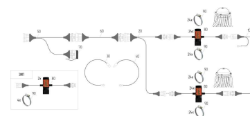
ЕТВ-6000000127, 66500686 Базовый комплект электроники СКИФ-38 с 05.2025
