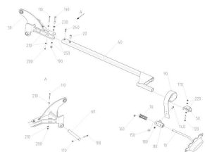
ЕТВ-6000000253, Гидрооборудование системы управления
