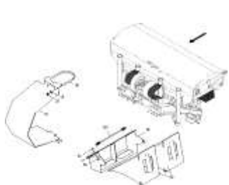
ЕТВ-0000010545, Задняя часть DMC 6000 L Аксессуары (2)
