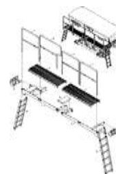
ETB-0000003148, Погрузочная площадка Primera DMC 6000 л (1)
