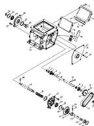
ЕТВ-0000003121, Дозатор 12000-2C лев./прав. (1)
