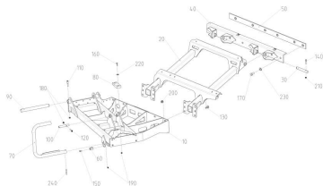
ЕТВ-6000000241, Рама правая
