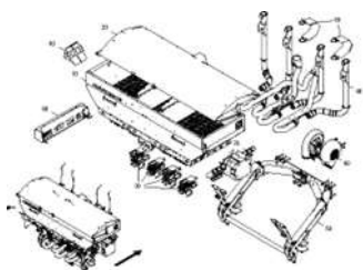
ЕТВ-0000010464, Задняя секция DMC 6000 L электрическая
