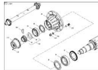
ЕТВ-0000003093, Ось без тормозов, (AM5ZA100P001)
