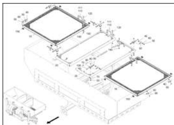
ЕТВ-0000005538, Контейнер 6000 л, Зибросте (03.2021- 10.2023)
