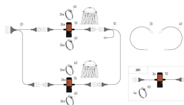
ЕТВ-6000000228, 66500362 Система контроля высева семян для DMC 9000 и 12000 с 48 сошниками с СКИФ-28 в базе (опция) до 05.2025
