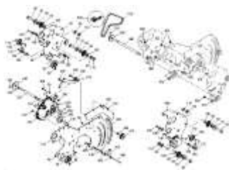
ЕТВ-0000007697, Редуктор агрегата удобрения 6000 л
