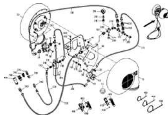
ЕТВ-0000005584, Двойной вентилятор
