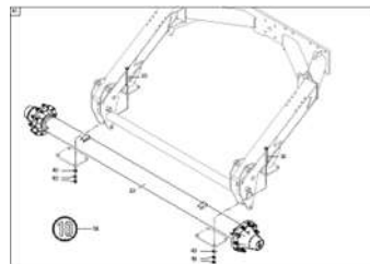
ЕТВ-0000008550, Ходовой мост 3300
