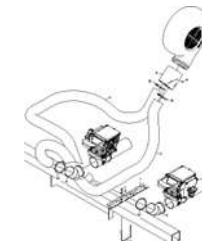
ЕТВ-0000003120, Подающая линия посевной материал удобрение (3)
