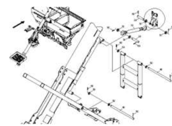
ETB-0000003179, Загрузочный шнек 6000L VM (7) / монтажные детали подшипник
